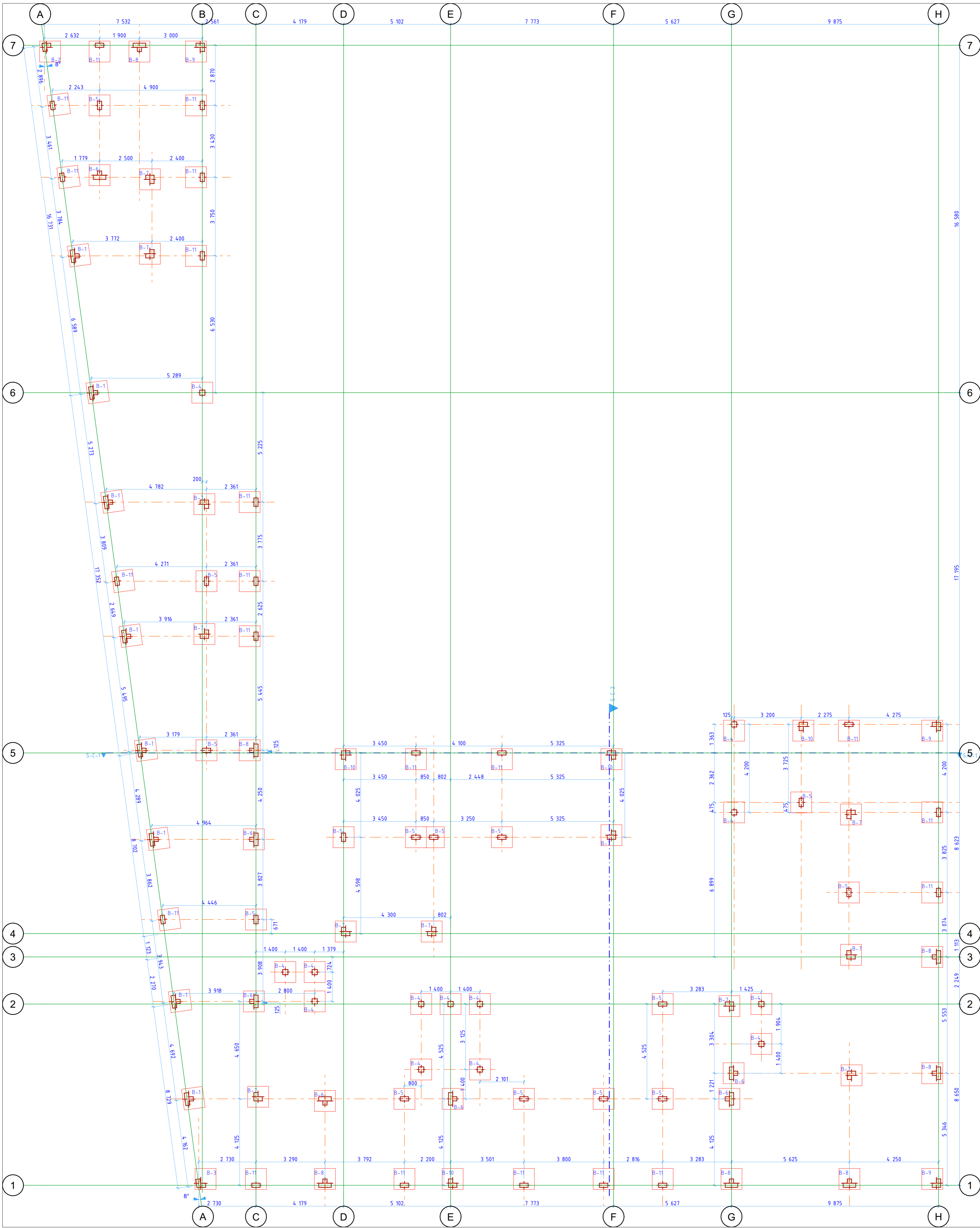
1. BASEMENT DIMENSIONS 1:100
